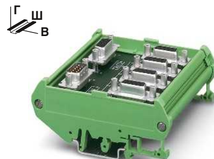
Т-образный разветвитель RS-485 (6-кратный), Разъем D-SUB
