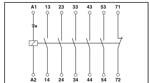
Реле сопряжения с принудительным замыканием и размыканием, 5 замыкающих и 1 размыкающий контакт
