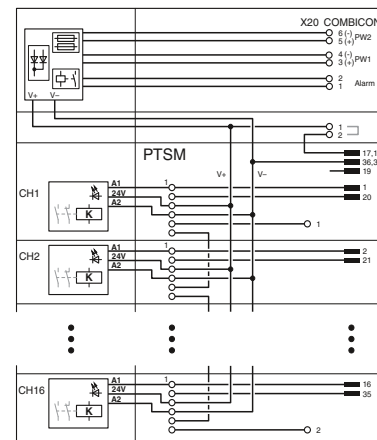
Схема соединений TC-2D37SUB-DO16-F&G-AR-UNI
