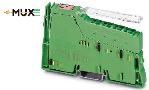
2 релейных выхода, 5-50 В перем. тона, 5-120 В пост. тона
