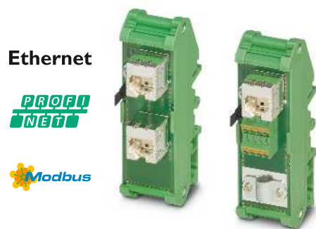
Мини-патч-панель с различными вариантами соединения
