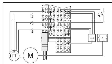
с интерфейсом инкрементального датчика или интерфейсом SSI для датчика абсолютных значений
