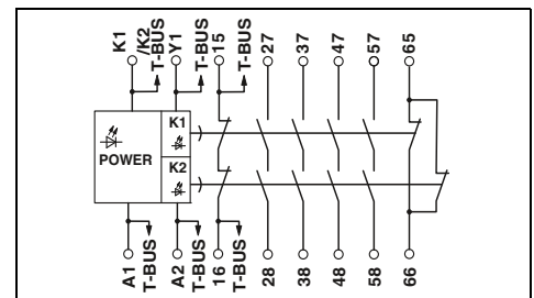
Модуль расширения с контактами с выдержкой времени на размыкание (установленное время 2 секунды)
