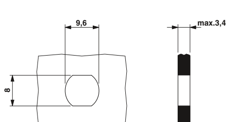
Чертёж отверстия для проходного монтажа разъёма B-FOC
