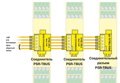
Соединители TBUS обеспечивают поперечное соединение между модулями.
