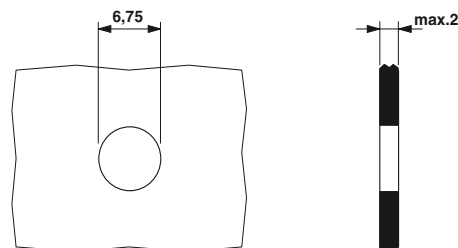
Чертёж отверстия для проходного монтажа разъёма F-SMA
