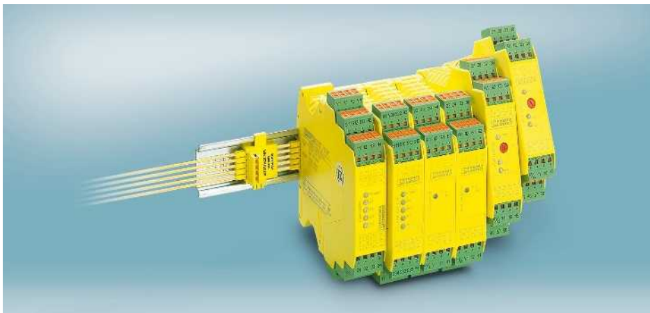
Соединители TBUS обеспечивают поперечное соединение между модулями.
